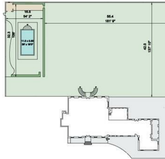
SITEPLAN
